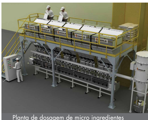
Planta de dosagem de micro ingredientes
